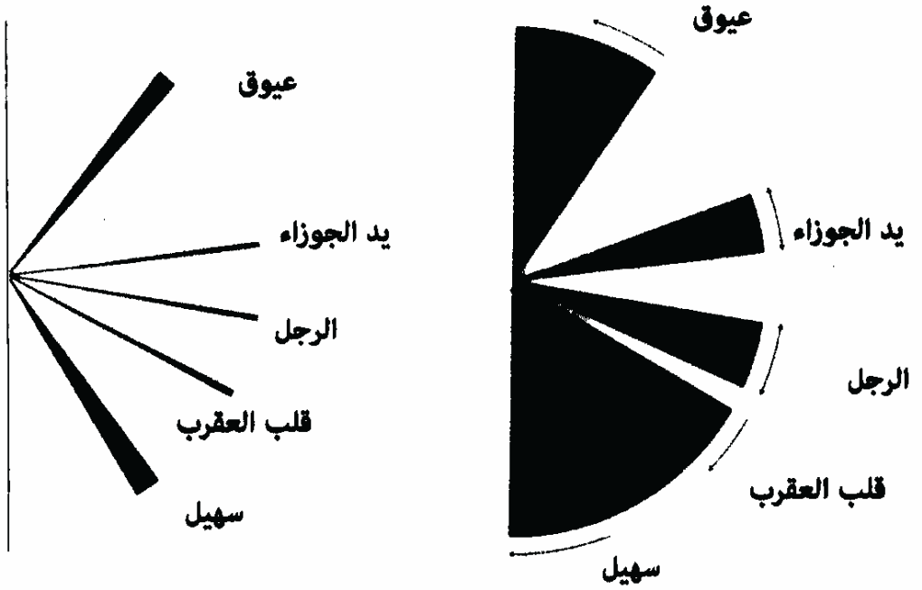
الشكل (69): مجال سمت الشروق لنجوم تحيط بخط الاستواء (يسار). ونجوم بين خطي عرض 30 و70 درجة شمالا.
